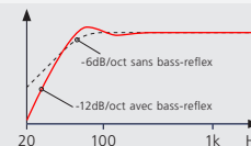
Les systèmes bass-reflex s'offrent un rajout de basses moyennes au prix de pertes dans les extrêmes ces basses factices sont mal contrôlées par l'ampli.
