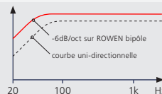
Cette technologie bipolaire ROWEN à basses actives autorise un boîtier clos (acoustic suspension) sans les inconvénients des systèmes bass-reflex.
