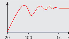
Les haut-parleurs uni-directionnels traditionnels sont à peu près linéaires à plus de 2m de la paroi.
